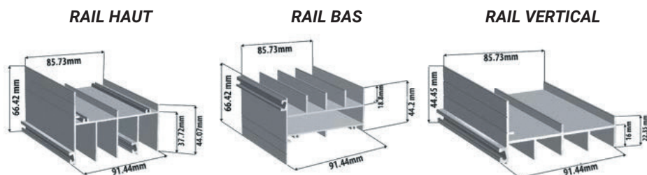
Cadre 4 rails (cadre 2 rails : cotes identiques sauf largeur : 49 mm au lieu de 91,44 mm)
